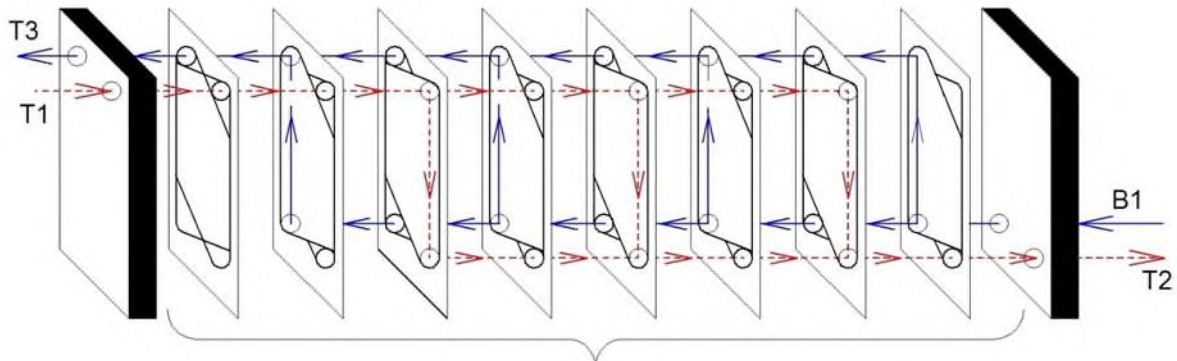
Рисунок А.2 - Компоновка пластин одноходового теплообменника с расположением патрубков с разных сторон теплообменника
