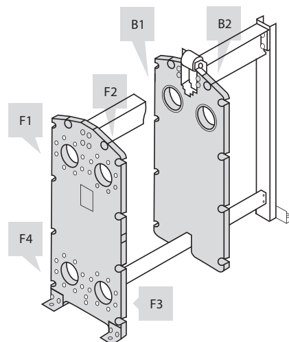
Рисунок E.2 - Расположение портов моноблочного теплообменника двухступенчатой системы ГВС
