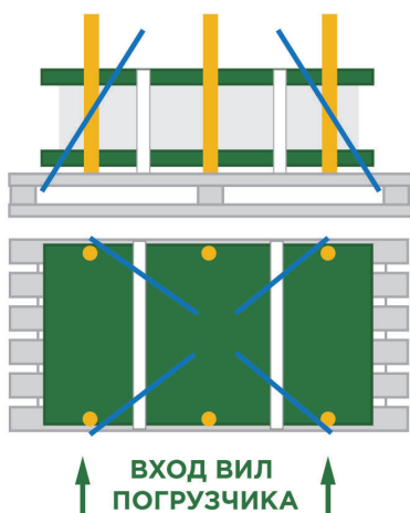
Рисунок А.2 - Схема строповки теплообменника без поддона
