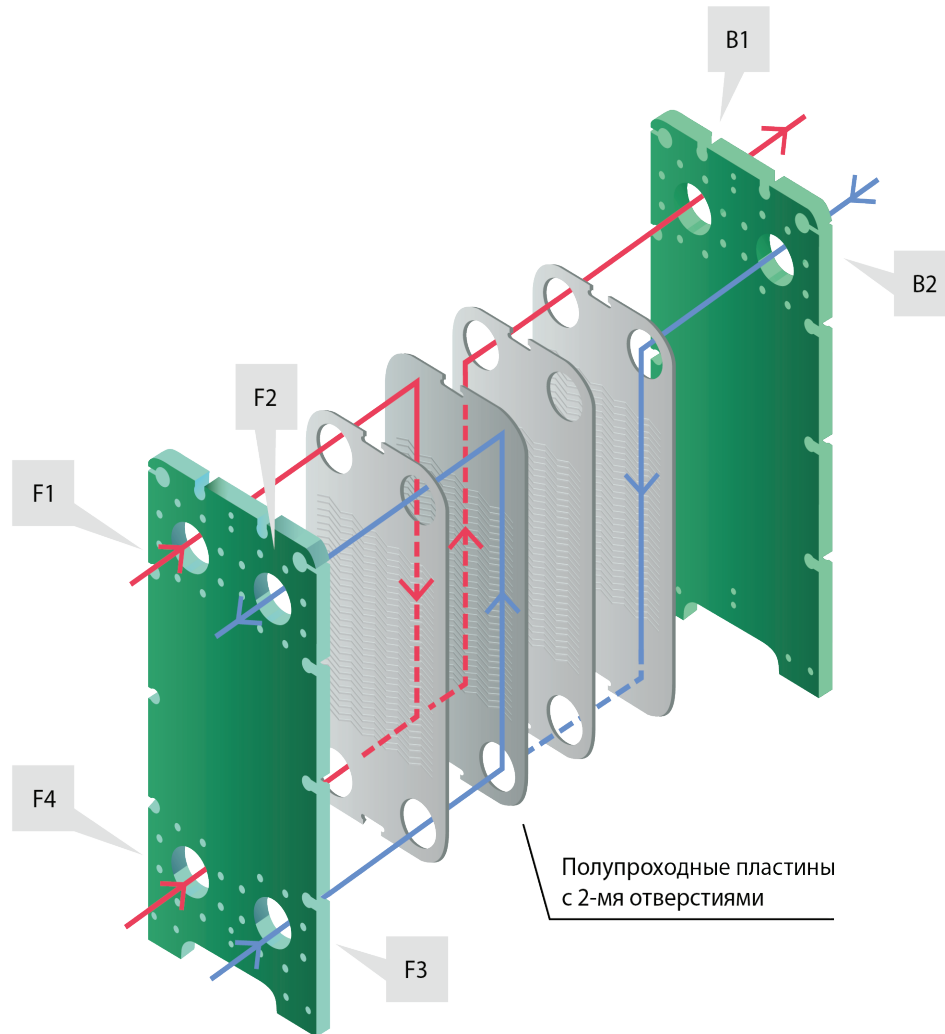
Рисунок Е.1 – Расположение 6-ти портов на передней (F) и задней (B) плитах
