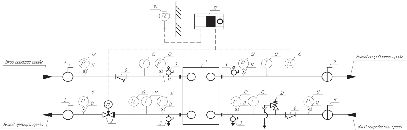
Рисунок Б.1 – Справочная схема обвязки теплообменника вода – вода
