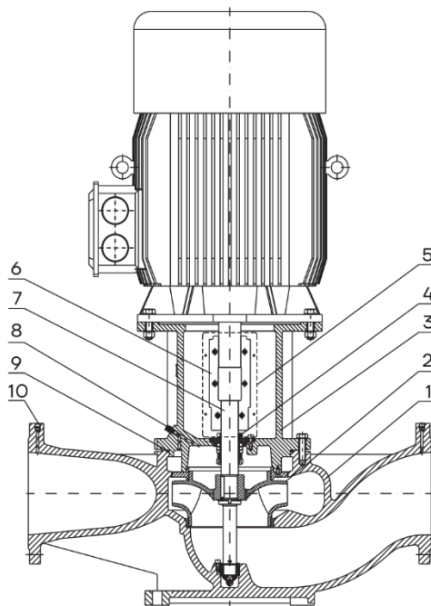
Рис. 2 Вид в разрезе TD200-TD250
