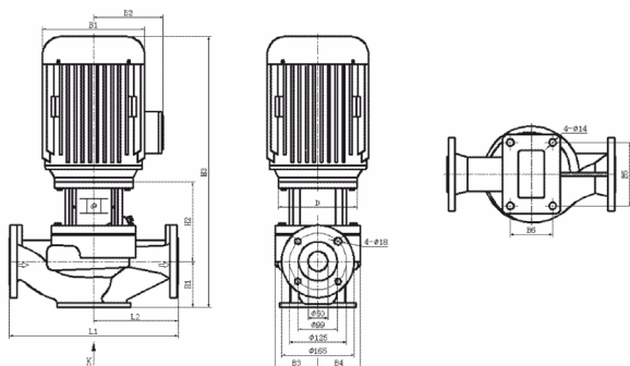
Рис. 20е. Габаритно-присоединительные размеры модели TD50-8(I)/2, TD50-12,5(I)/2
