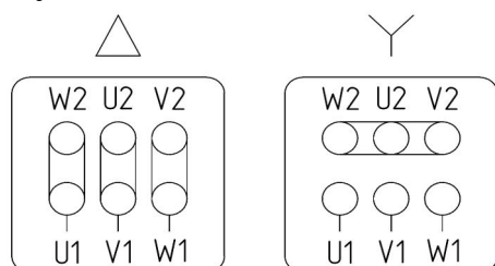
Рисунок 4. Схема подключения фаз электропитания.
